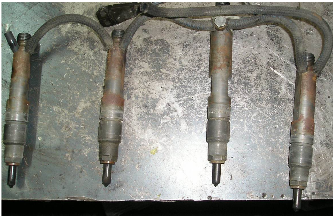
Εικόνα 8-8 Αρχική κατάσταση εγχυτήρων καυσίμου του VW Golf
