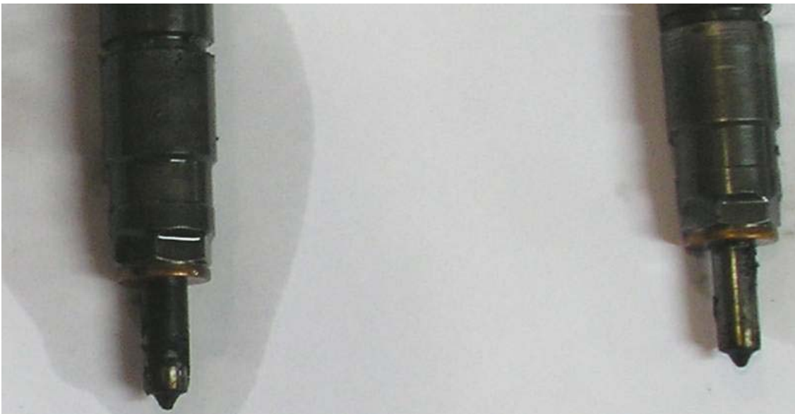
Εικόνα 8-12 Εγχυτήρας καυσίμου Renault Laguna μετά την εφαρμογή των μιγμάτων βαμβακελαίου-diesel
